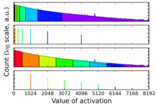
Figure 2: 로그 값을 이용한 Quantization의 예
