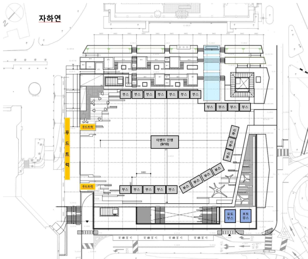
<부스 배치도>
